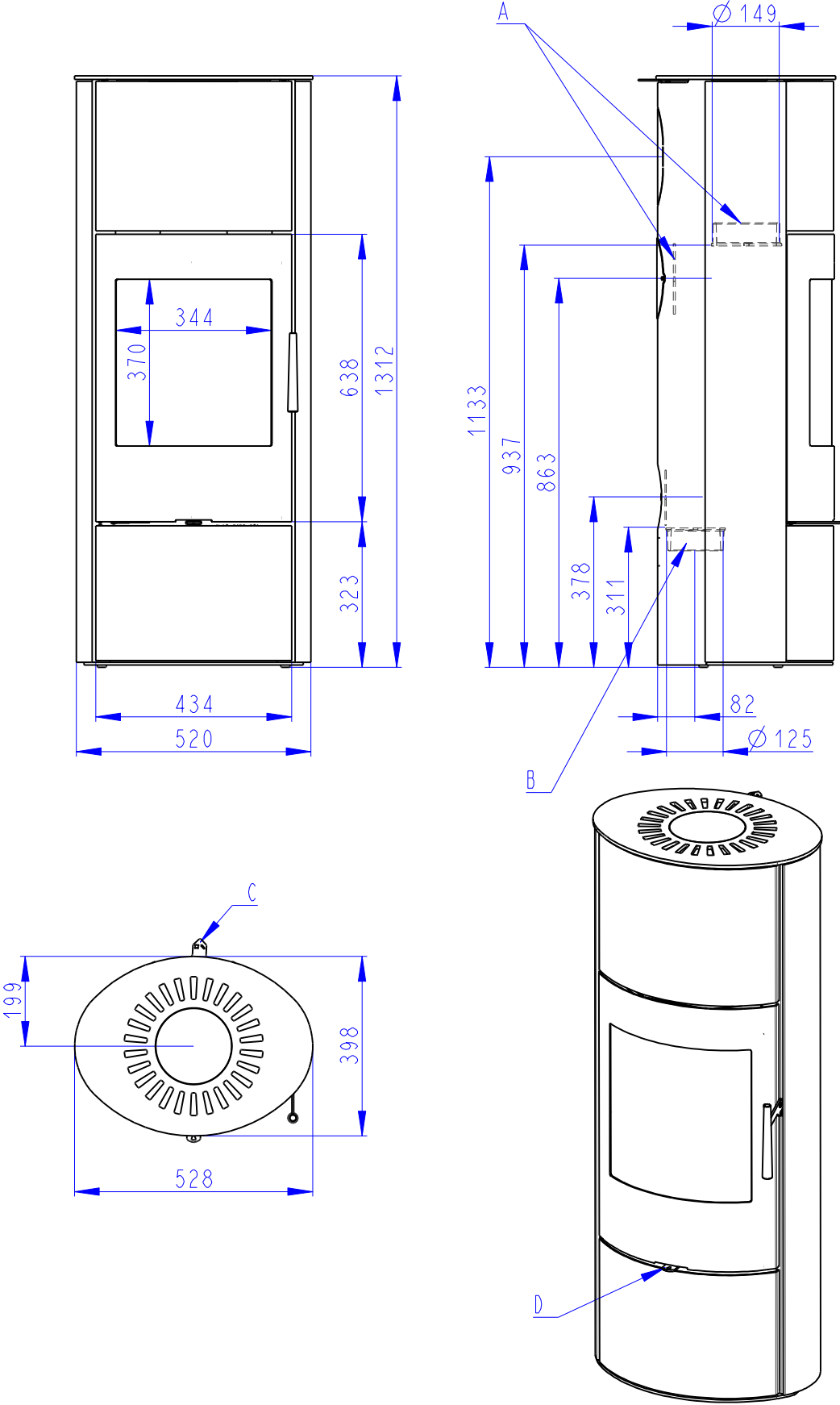
EVORA AKUM - Rozměrový náčrt, Rozmerový náčrt, Schemat wymiarowy, Размерный эскиз
